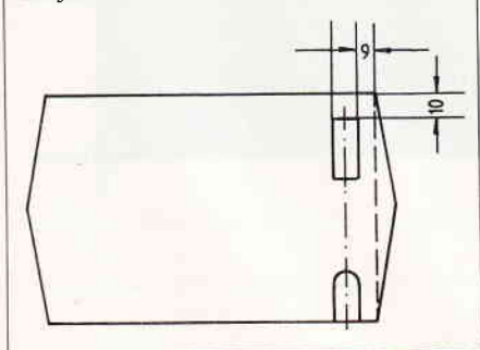
Abb. 11: Maßskizze der Gehäuserückwand
