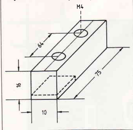
Abb. 10: Maße der Halteleiste für Trafo
