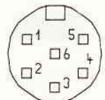
Die Videobuchse (Pinout)
