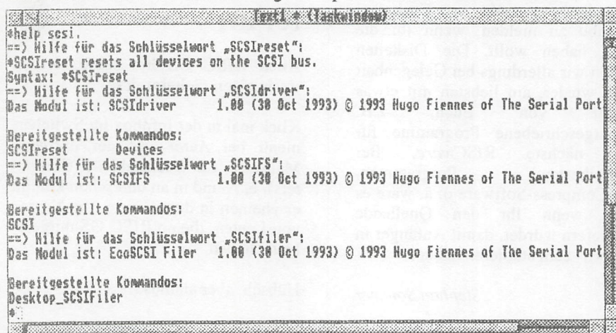
Die CLI-Befehle des EcoSCSI-Controllers
